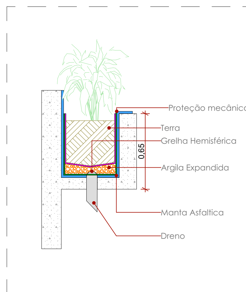
Detalhe Floreira 1:20
