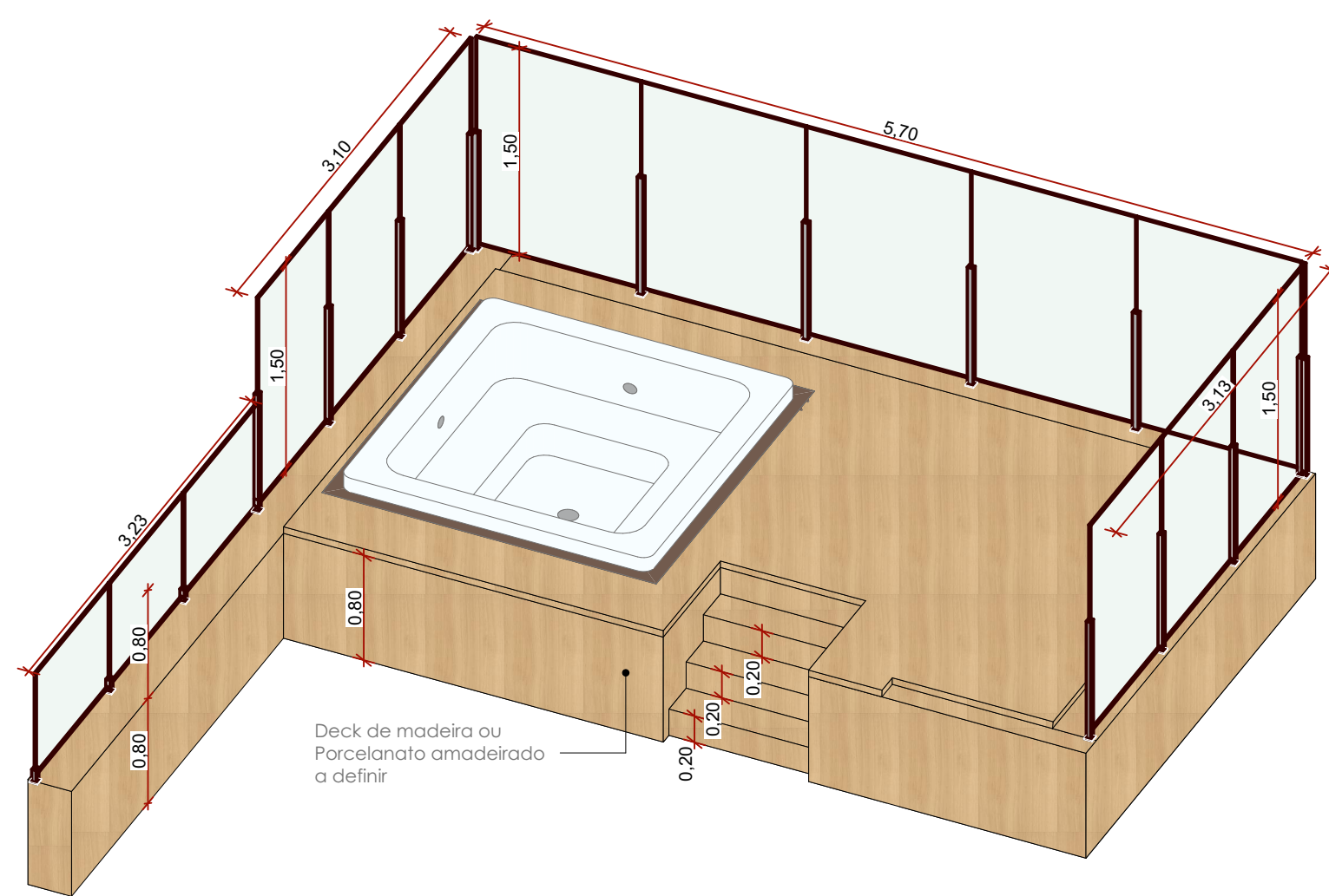
ISOMETRICA SPA 1:50
